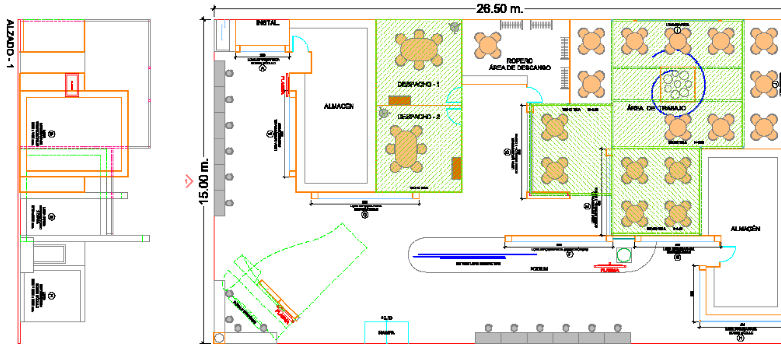
PLANTA DE DISTRIBUCIÓN ESCALA 1/100
